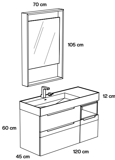
Ref. CA1060412I Bajo lavabo compacto decorativo seno izquierdo 2 cajones y puerta con hueco (Under basin compact module with left sink, 2 drawers and door with hole) 120 x 60 x 45 cm
